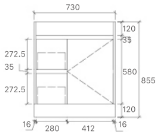
SY05-750L Size: 730x450x855mm
