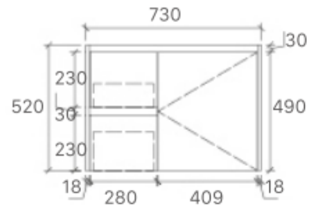
WH76-750L Size: 730x455x520mm
