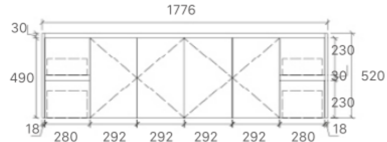
WH76-1800 Size: 1776x455x520mm
