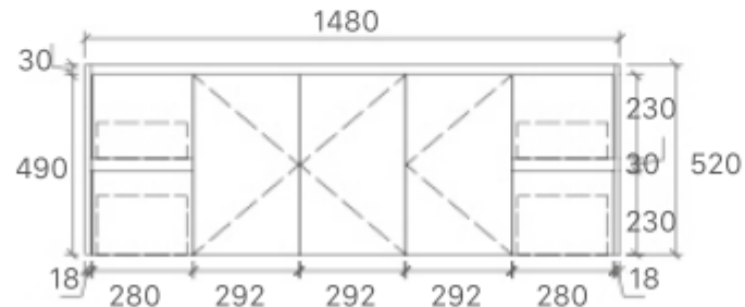
WH76-1500 Size: 1480x455x520mm
