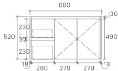
WH76-900L Size: 880x455x520mm
