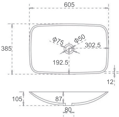
■ URBAN SI-A06G-605 or SI-A06-605 Color: Gloss White or Matt White Size: 605x385x105mm
