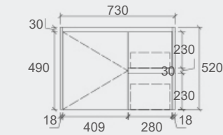
WH76-750R Size: 730x455x520mm
