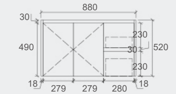
WH76-900R Size: 880x455x520mm
