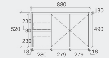
WH76-900L Size: 880x455x520mm
