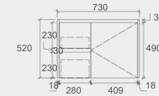
WH76-750L Size: 730x455x520mm
